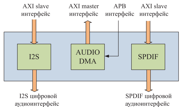
Рис. 4. Структурная схема аудиоконтроллера
