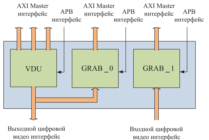
Рис. 3. Структурная схема подсистемы ввода/вывода видеоданных
