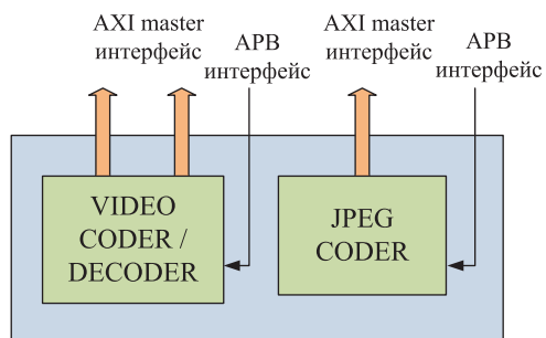
Рис. 5. Структурная схема подсистемы кодирования и декодирования видеоизображения
