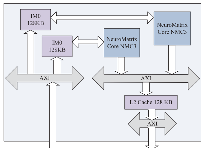
Рис. 2. Структура процессорной подсистемы ЦОС СБИС МИВЭМ
