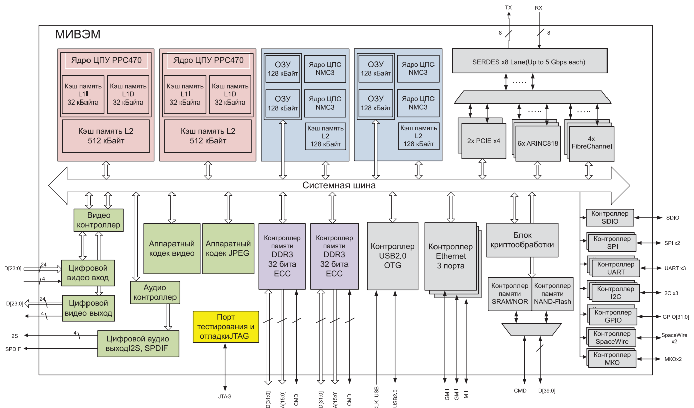
Рис. 1. Структурная схема СБИС МИВЭМ
