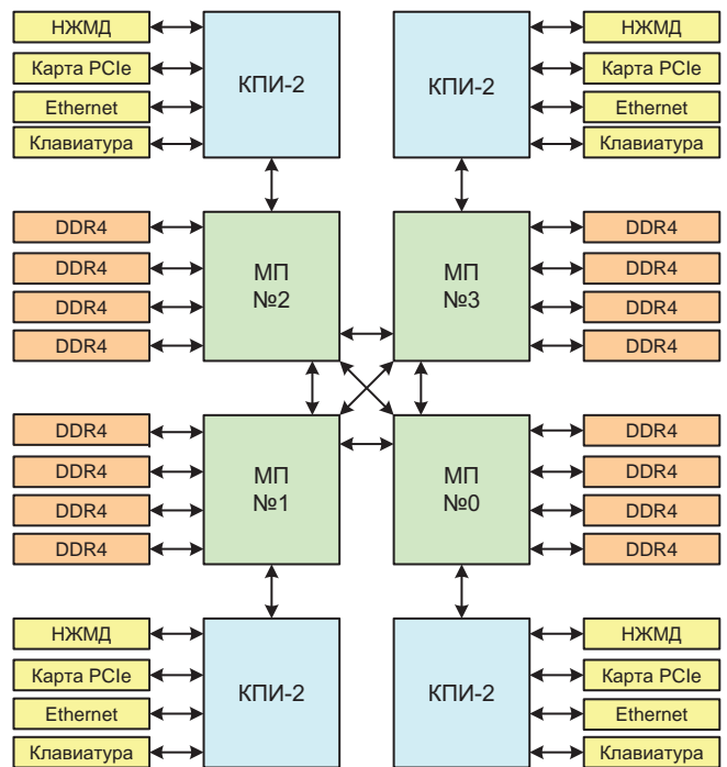
Рис. 2. Схема вычислительной системы на основе МП «Эльбрус-8С»
