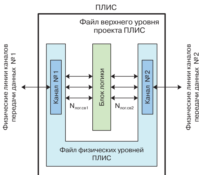
Рис. 3. Схема микроархитектурных связей в МП «Эльбрус-8С»
