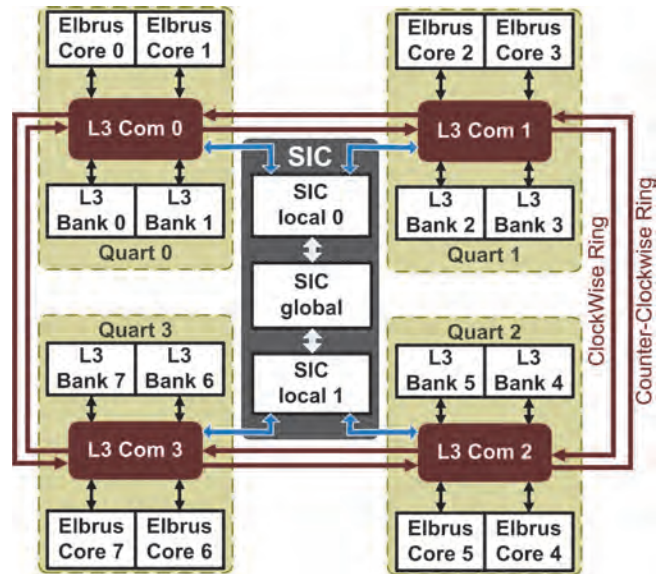
Рис. 1. Схема микроархитектурных связей в МП «Эльбрус-8С»
