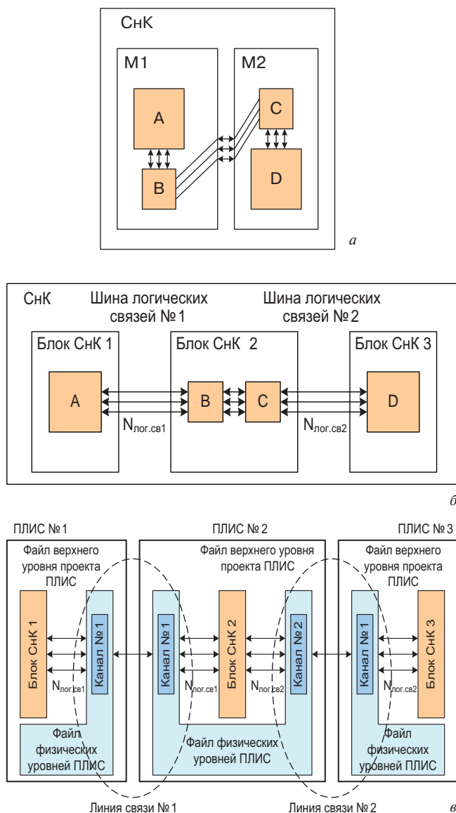
Рис. 10. Схема распределения единой RTL-модели МП в системе эмуляции из ПЛИС: а) схема RTL-модели, б) представление блоков RTL-модели МП после деления, в) представление блоков RTL-модели МП в ПЛИС распределенной системы эмуляции
