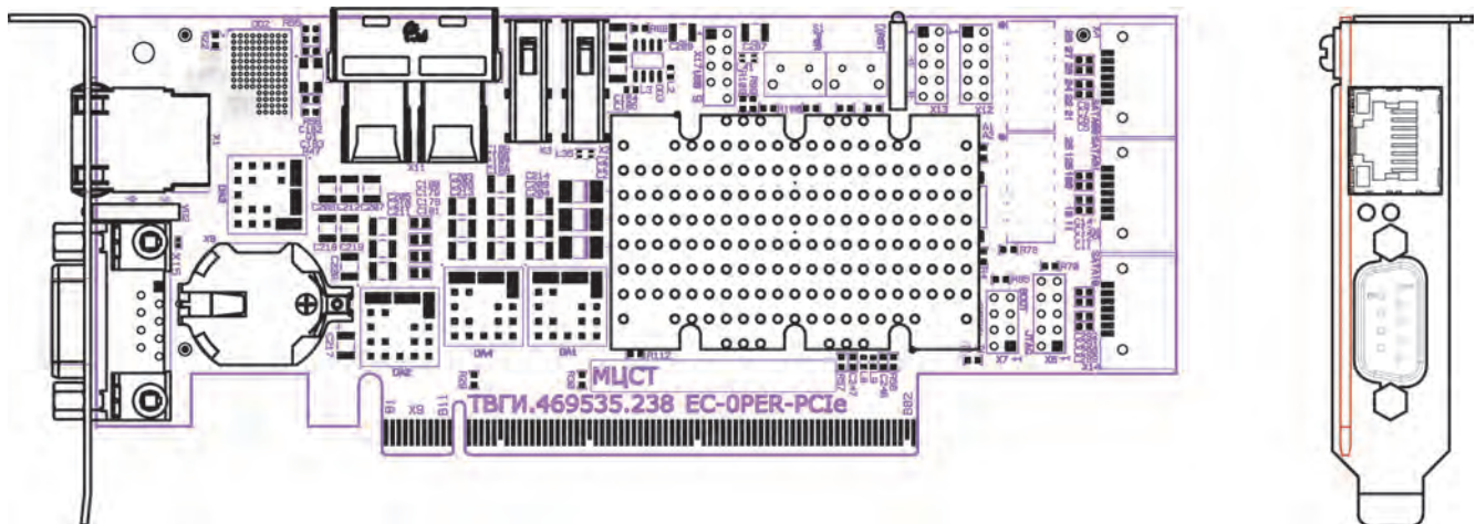
Рис. 7. Карта расширения внешнего КПИ-2
