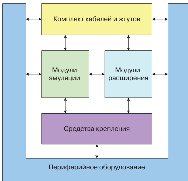
Рис. 4. Схема аппаратного состава масштабируемой системы эмуляции
