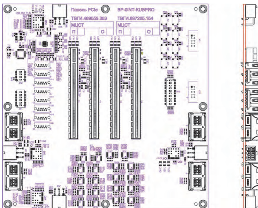
Рис. 6. Панель PCIe BP-01INT-KUBPRO
