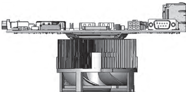
Рис. 5. Форм-фактор «КУБ-ПРО»: а) пример положения элементов модуля, б) 3D-модель модуля (вид сбоку)
