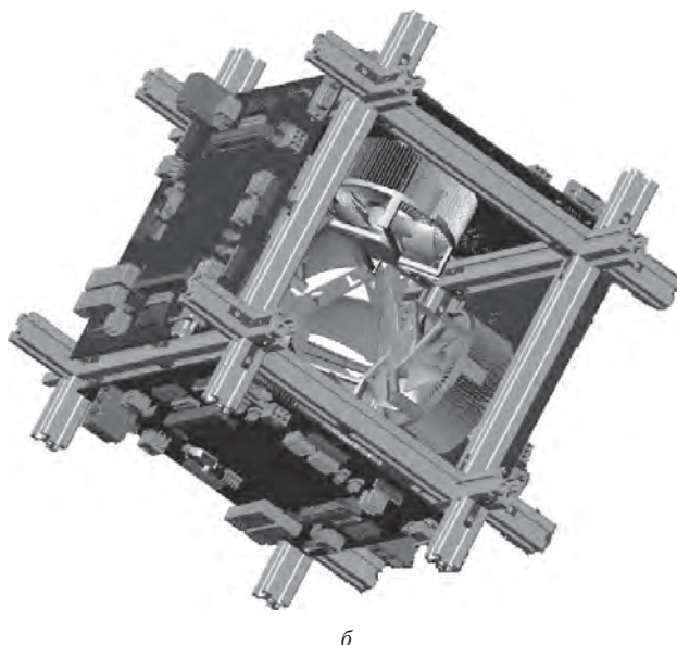
Рис. 9. 3D-модель каркаса: а) внешний вид каркаса, б) каркас с четырьмя модулями в форм-факторе «КУБ-ПРО»
