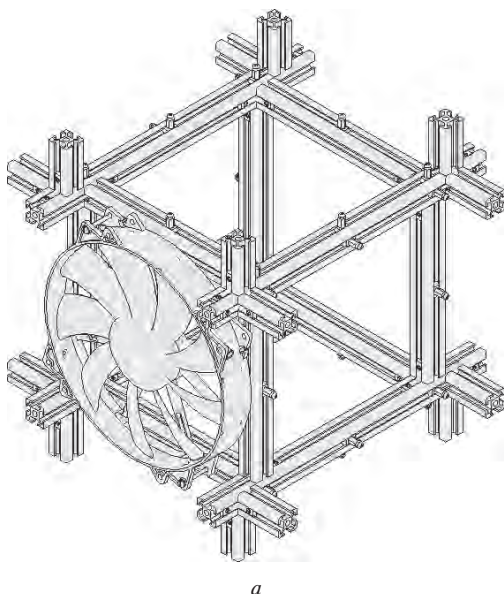
Рис. 9. 3D-модель каркаса: а) внешний вид каркаса, б) каркас с четырьмя модулями в форм-факторе «КУБ-ПРО»
