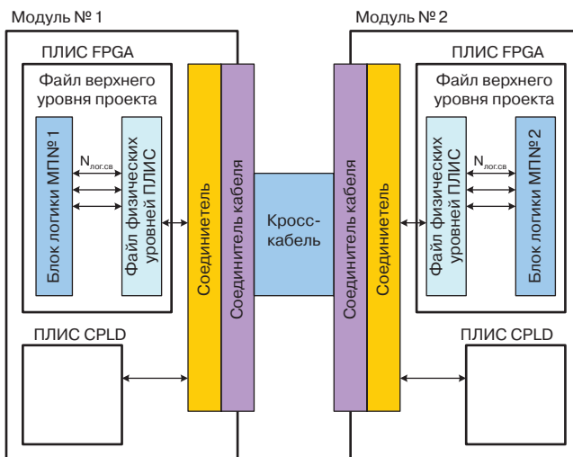
Рис. 8. Схема интерфейса прототипа
